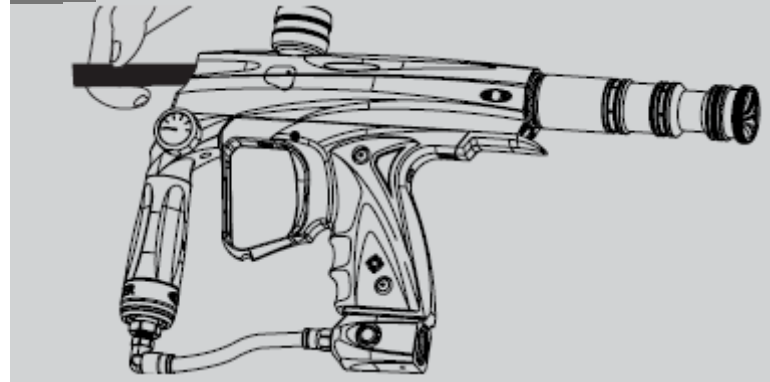
FIG.16 → ВЫТАЛКИВАНИЕ СБОРКИ ЗАТВОРА
