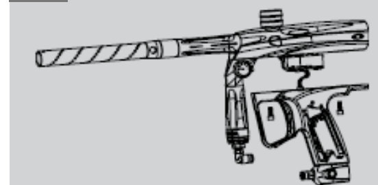
FIG.24 → ОТСОЕДИНЕНИЕ РАМКИ РУКОЯТКИ
