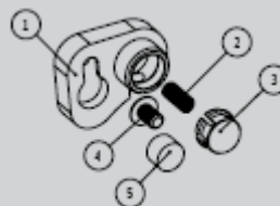
FIG.21 → СБОРКА БОЛ ДЕТЕНТА
